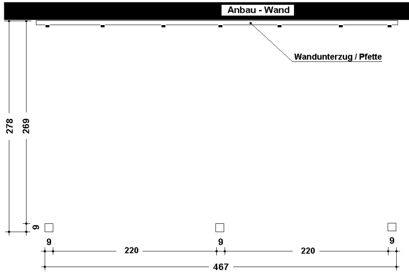
Pfostenplan
