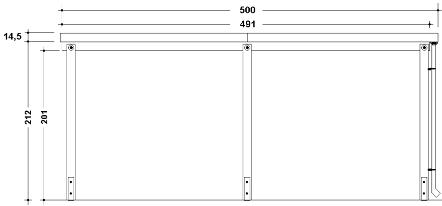
Seitenansicht
