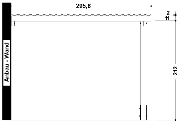
Schnitt
