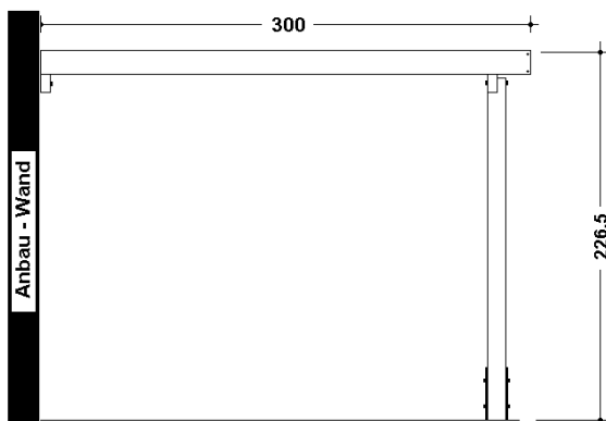
Vorderansicht
