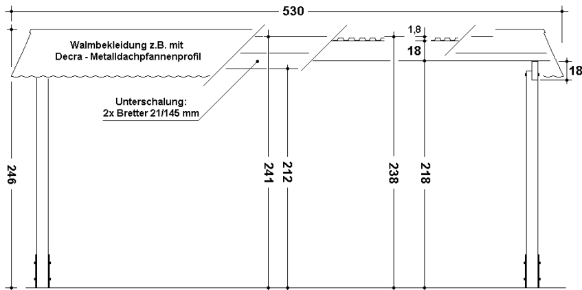
Vorderansicht / Schnitt
