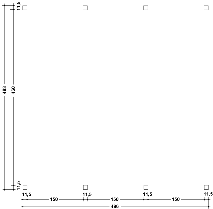
Pfostenplan
